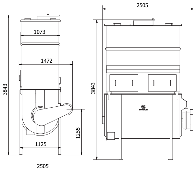
2 étages: mélangeur + bac de pré-mélange
