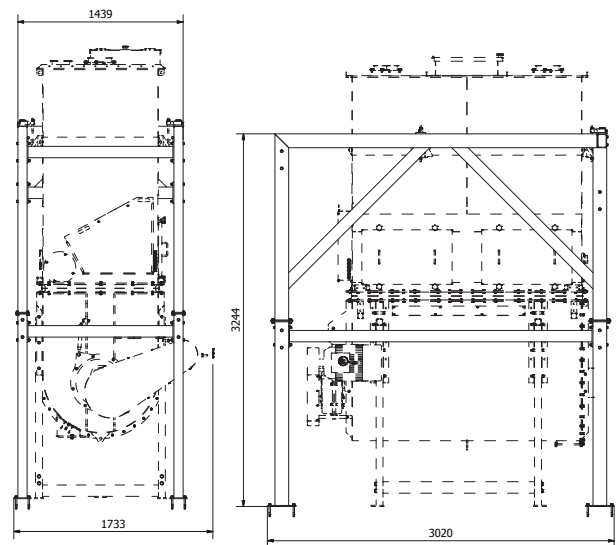
2 étages: support de bac de pré-mélange
