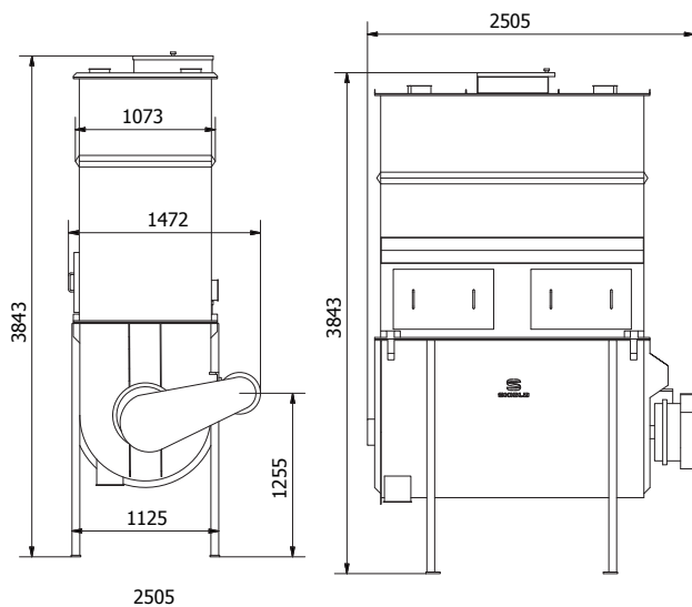
2-trins – blender + forbeholder
