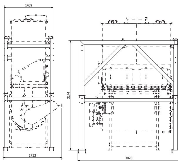
2-trins – blender + forbeholder + stativ
