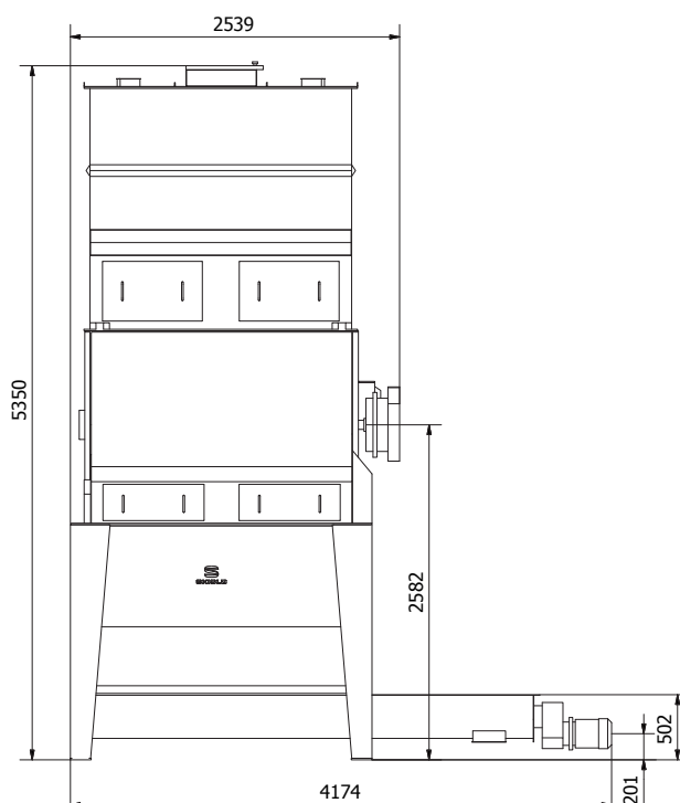
3-trins – blender + forbeholder + efterbeholder
